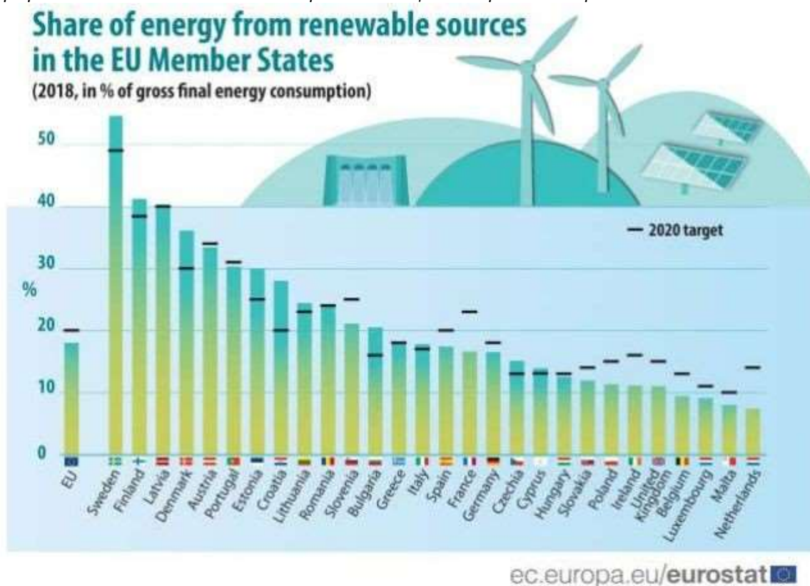
Графика на дела на възобновяема енергия към общото енергийно потребление в ЕС за 2018 година
